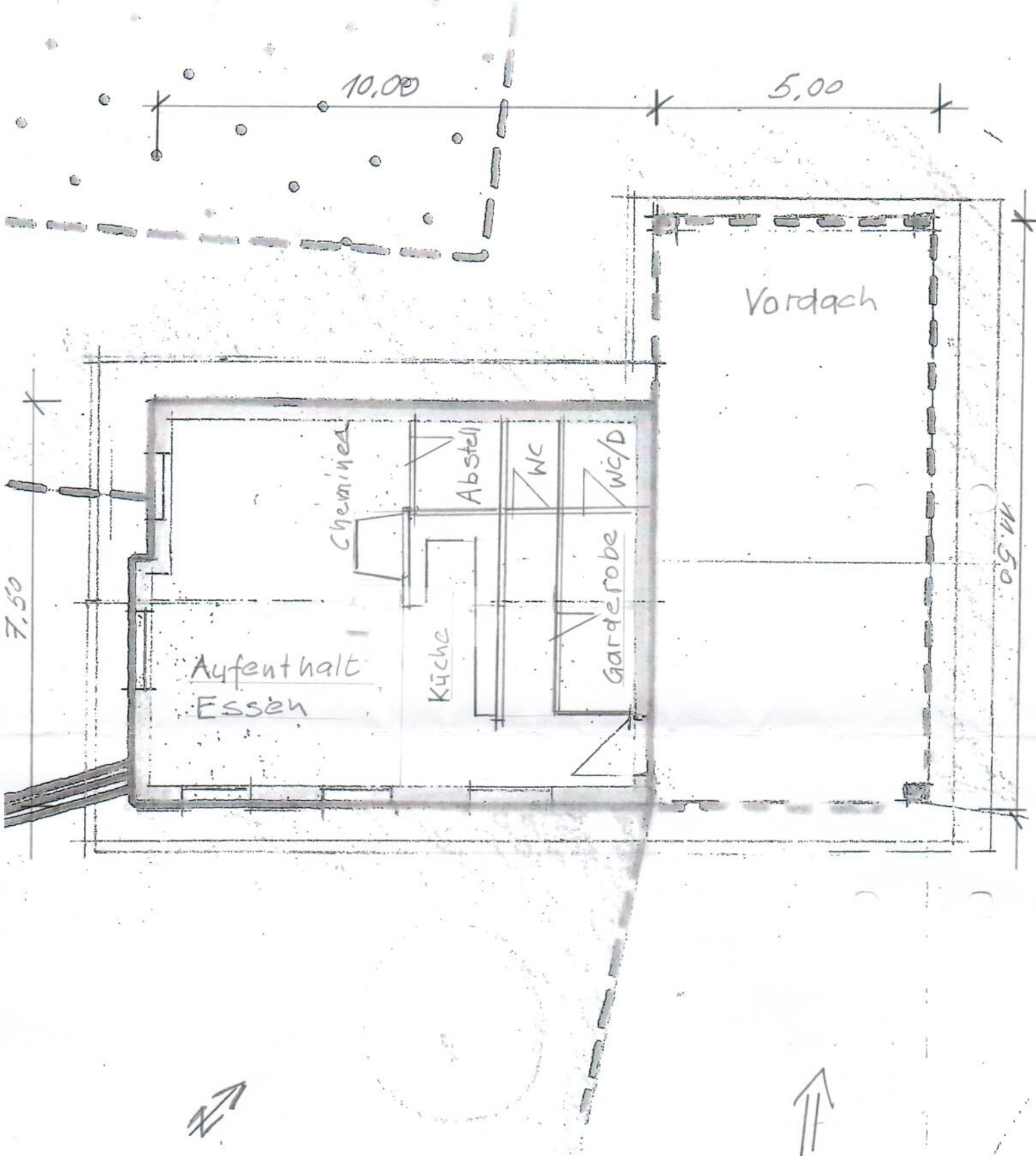
Beilage B Bestehendes Forsthaus Grundriss EG 1:100
